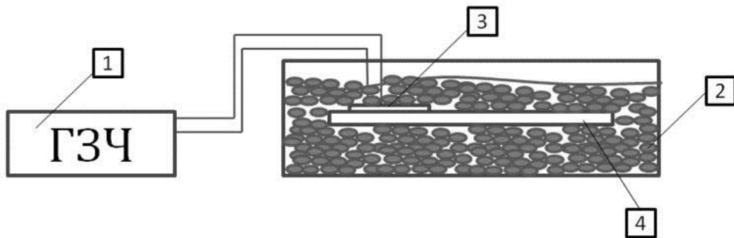
1 – генератор ЛЗ0; 2 – резервуар з робочим середовищем для вібраційної обробки; 3 – п'єзоелектричний датчик; 4 – зразок
